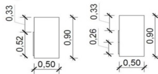
3 VISTAS LATERAIS
